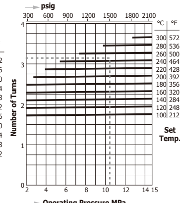
TBH82 - 150
