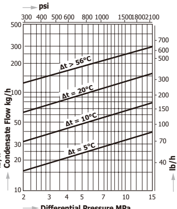
TBH82 - 150
