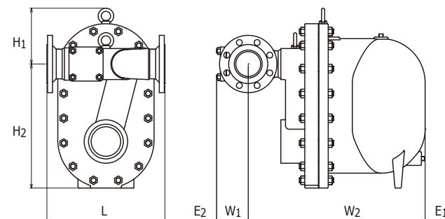
Dimensions GH70
