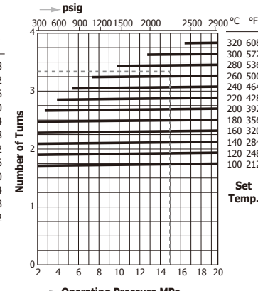
TBH82 - 200
