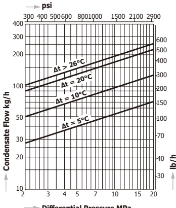
TBH81 - 200
