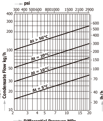
TBH82 - 200
